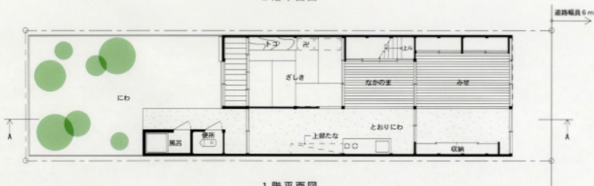
1階平面図
